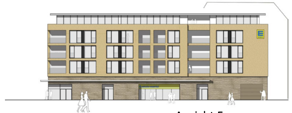
Ansicht Feuerseeweg
